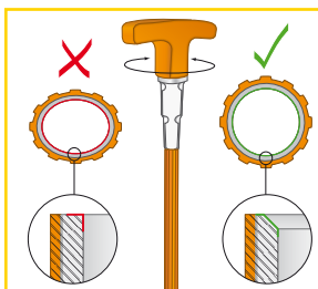
▲ Rohr kalibrieren und anfasen
